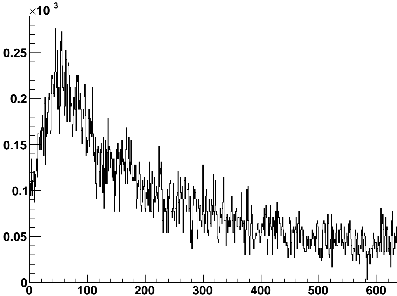
module_L6b_halfmodule_stereo_slot_sensor0 - Occupancy
