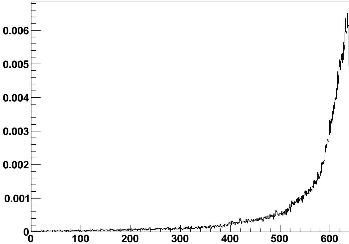
module_L2b_halfmodule_stereo_sensor0 - Occupancy
