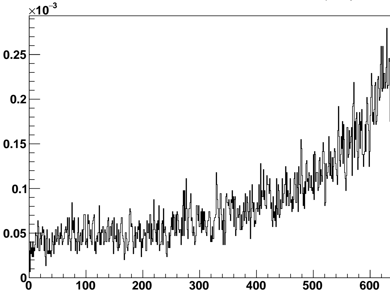
module_L6t_halfmodule_axial_slot_sensor0 - Occupancy
