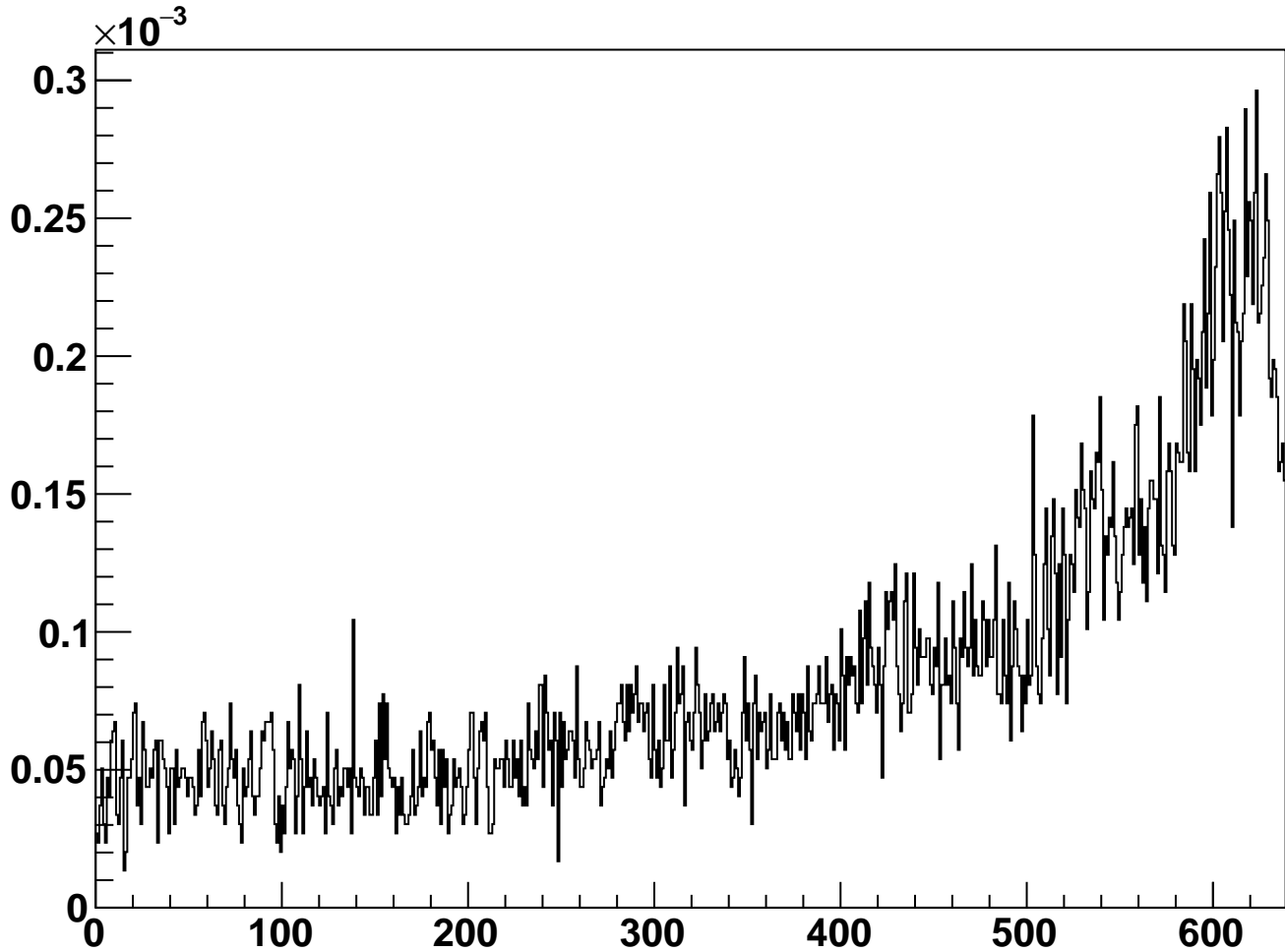
module_L6b_halfmodule_axial_slot_sensor0 - Occupancy
