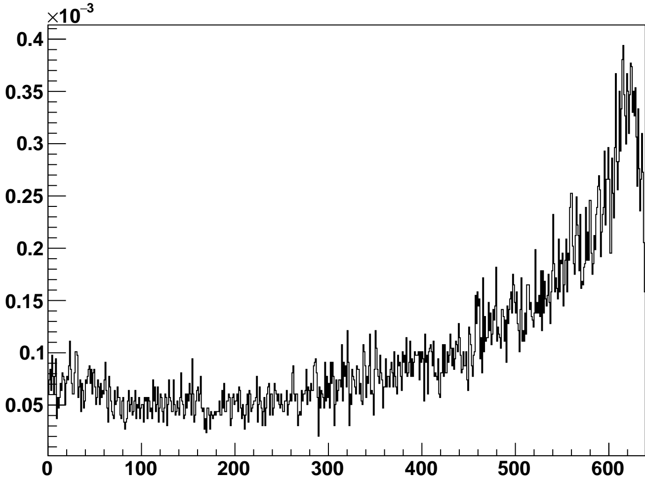
module_L5b_halfmodule_axial_slot_sensor0 - Occupancy
