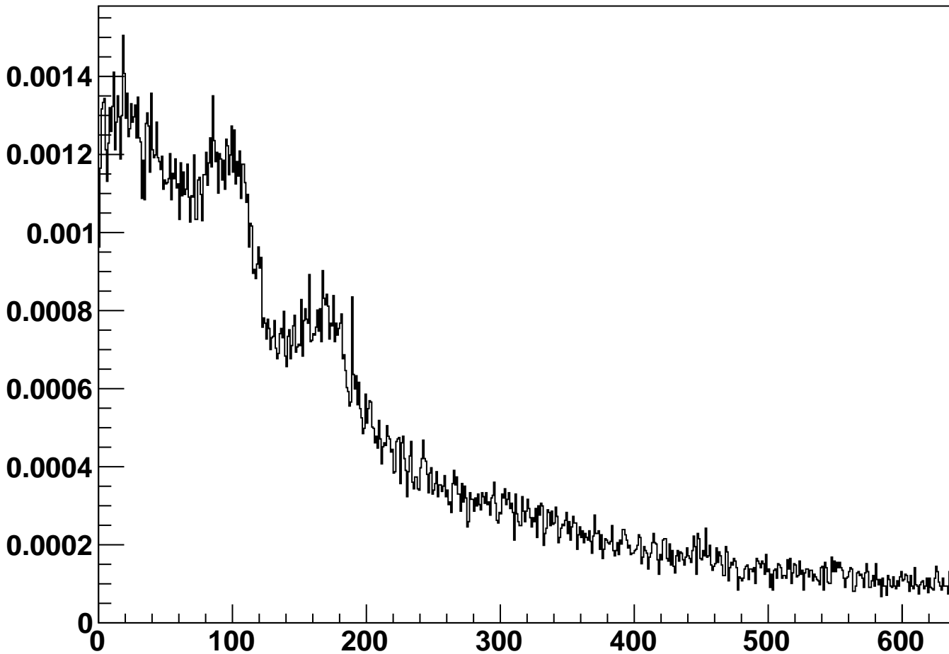
module_L6b_halfmodule_axial_hole_sensor0 - Occupancy
