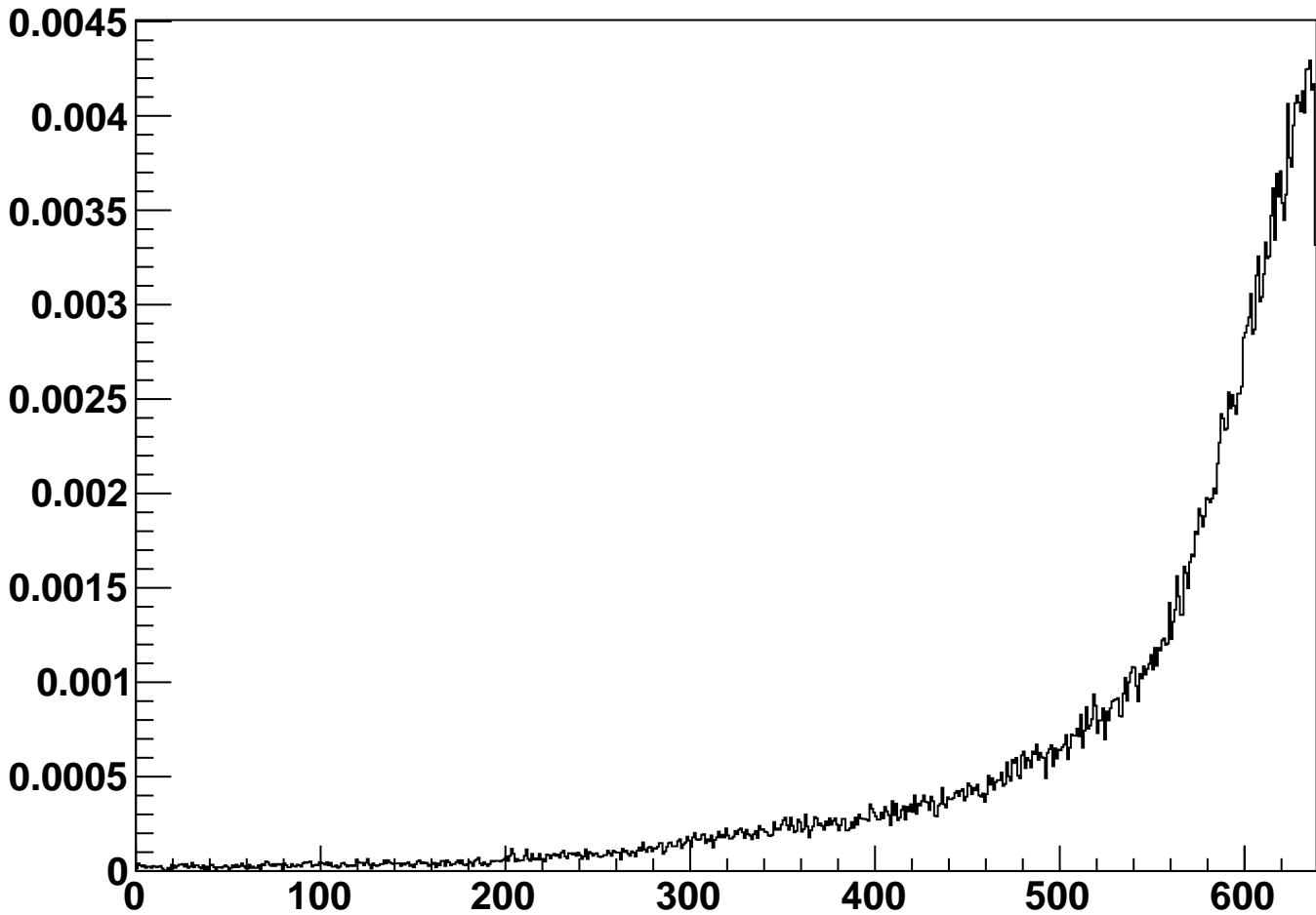
module_L3b_halfmodule_stereo_sensor0 - Occupancy
