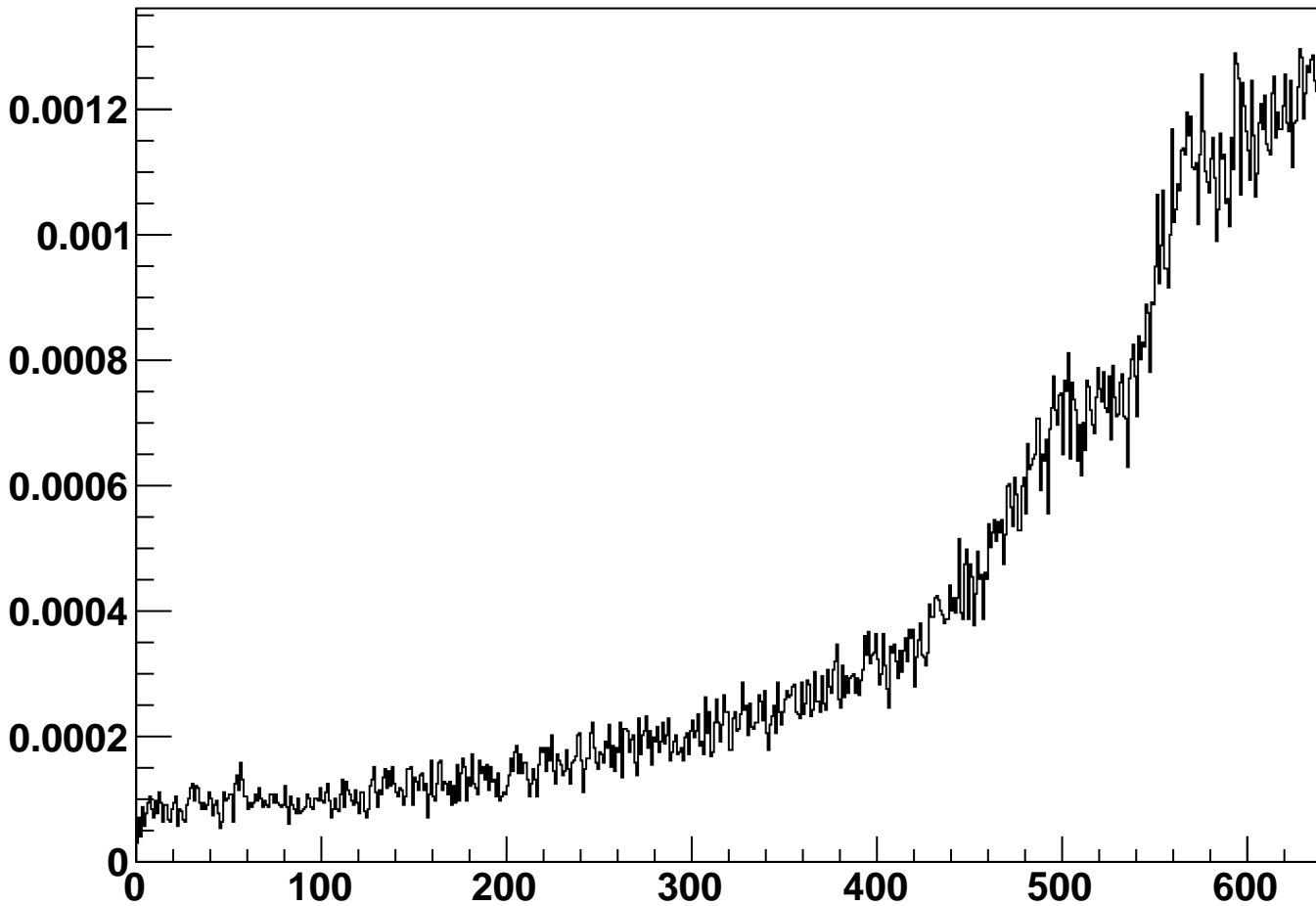
module_L6b_halfmodule_stereo_hole_sensor0 - Occupancy
