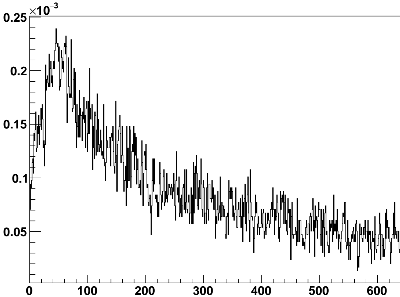
module_L6t_halfmodule_stereo_slot_sensor0 - Occupancy
