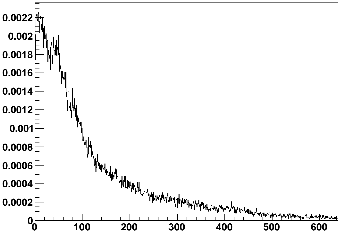
module_L4t_halfmodule_axial_hole_sensor0 - Occupancy
