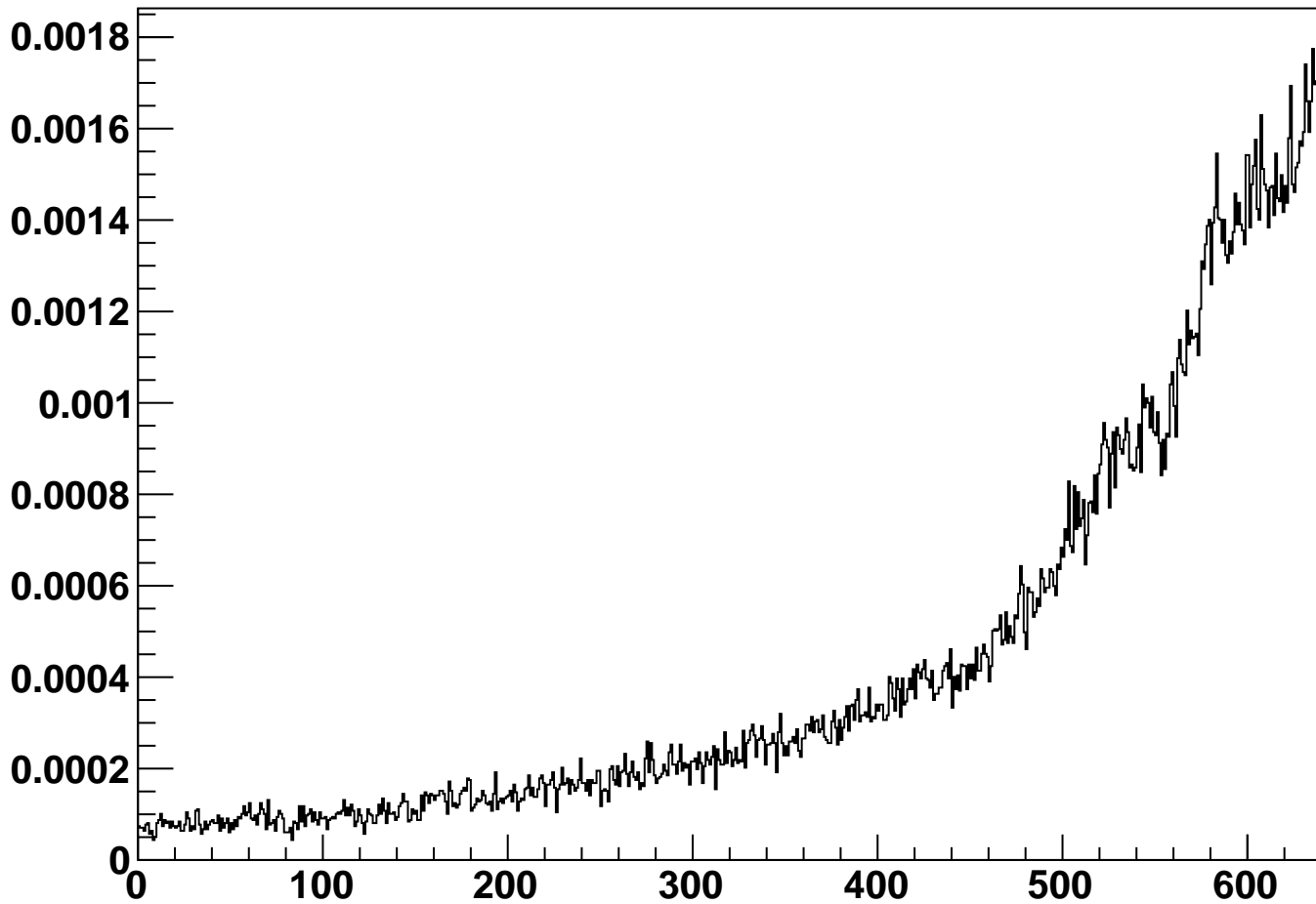
module_L5b_halfmodule_stereo_hole_sensor0 - Occupancy
