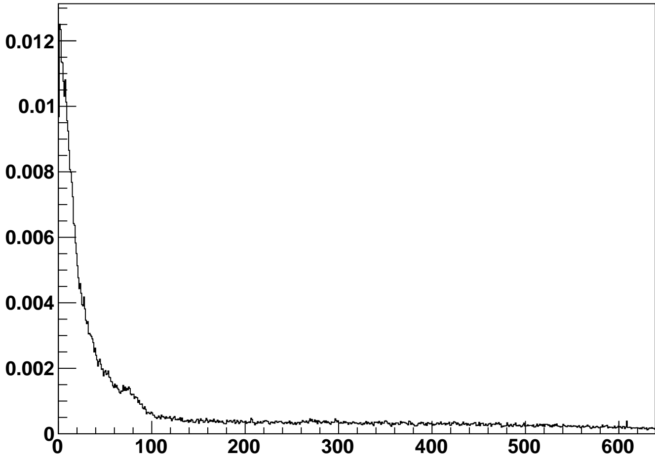
module_L1t_halfmodule_axial_sensor0 - Occupancy
