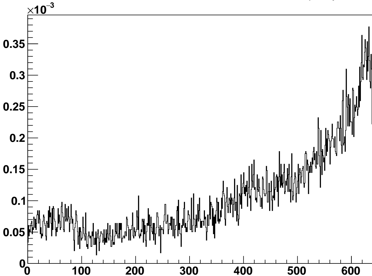
module_L5t_halfmodule_axial_slot_sensor0 - Occupancy
