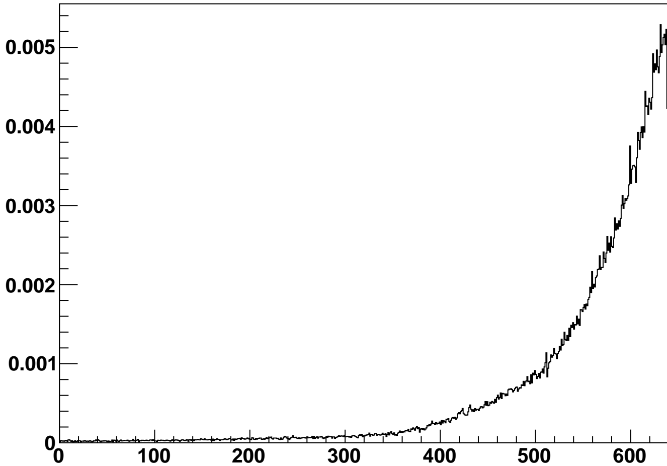
module_L3b_halfmodule_stereo_sensor0 - Occupancy
