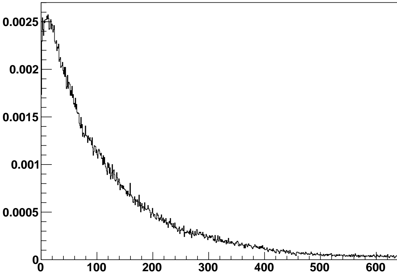
module_L4b_halfmodule_axial_hole_sensor0 - Occupancy
