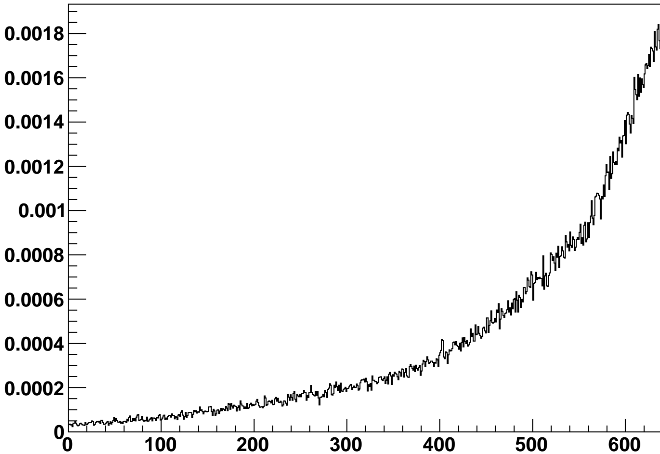
module_L5b_halfmodule_stereo_hole_sensor0 - Occupancy
