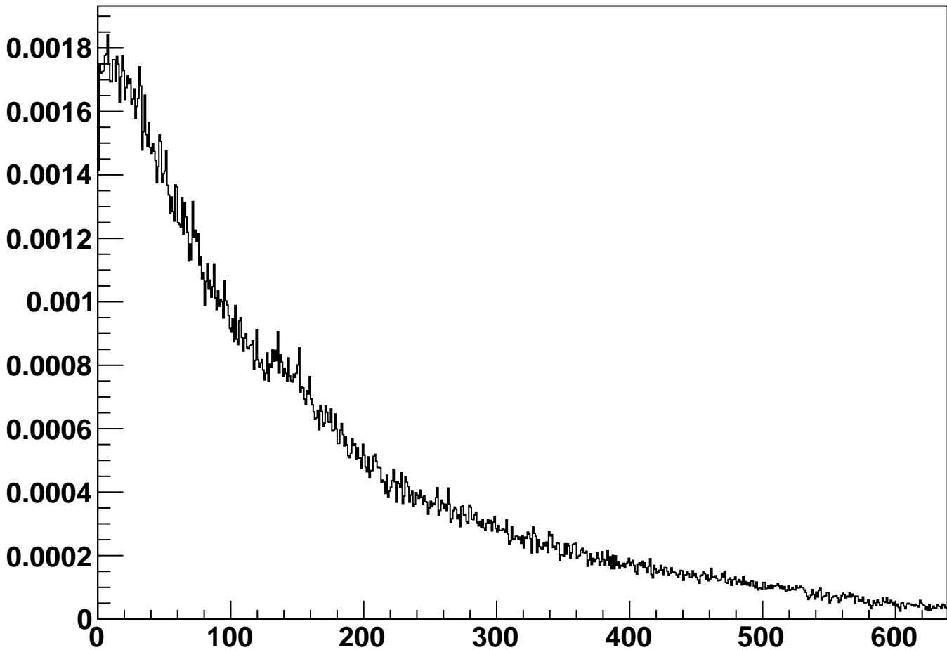
module_L5t_halfmodule_axial_hole_sensor0 - Occupancy
