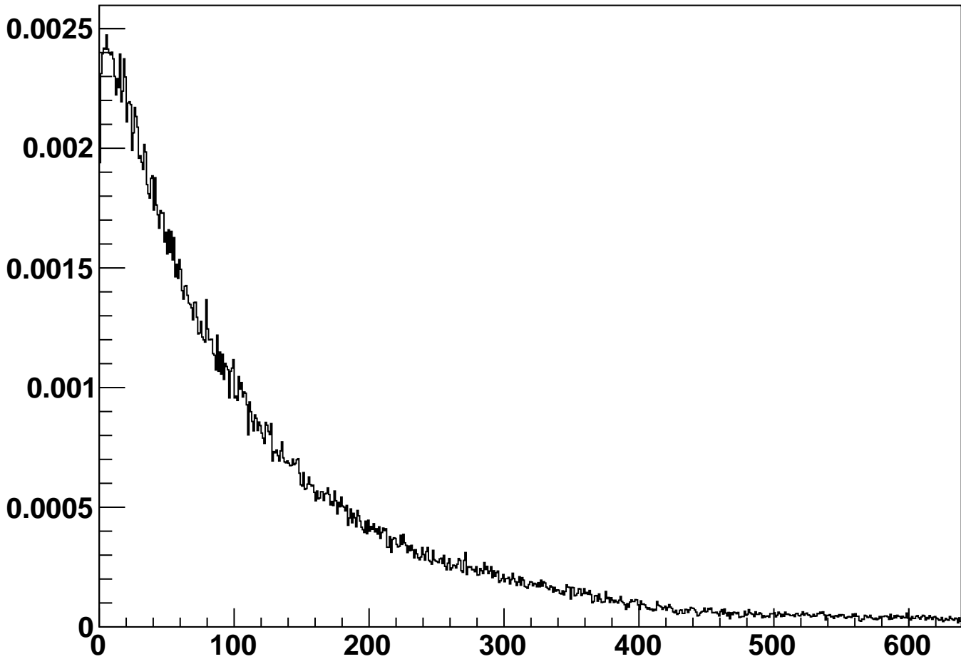
module_L4t_halfmodule_axial_hole_sensor0 - Occupancy
