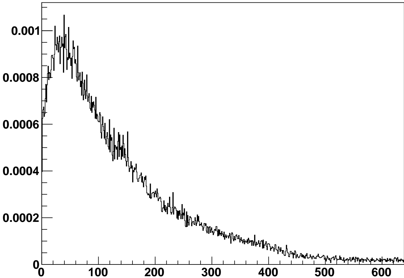
module_L4b_halfmodule_stereo_slot_sensor0 - Occupancy
