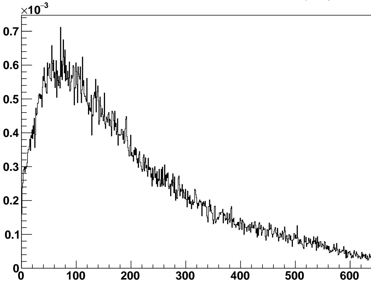
module_L5t_halfmodule_stereo_slot_sensor0 - Occupancy
