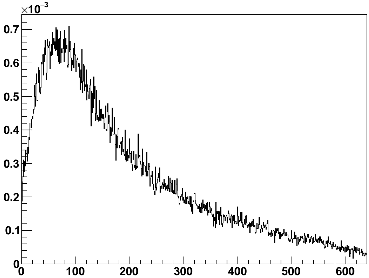
module_L5b_halfmodule_stereo_slot_sensor0 - Occupancy
