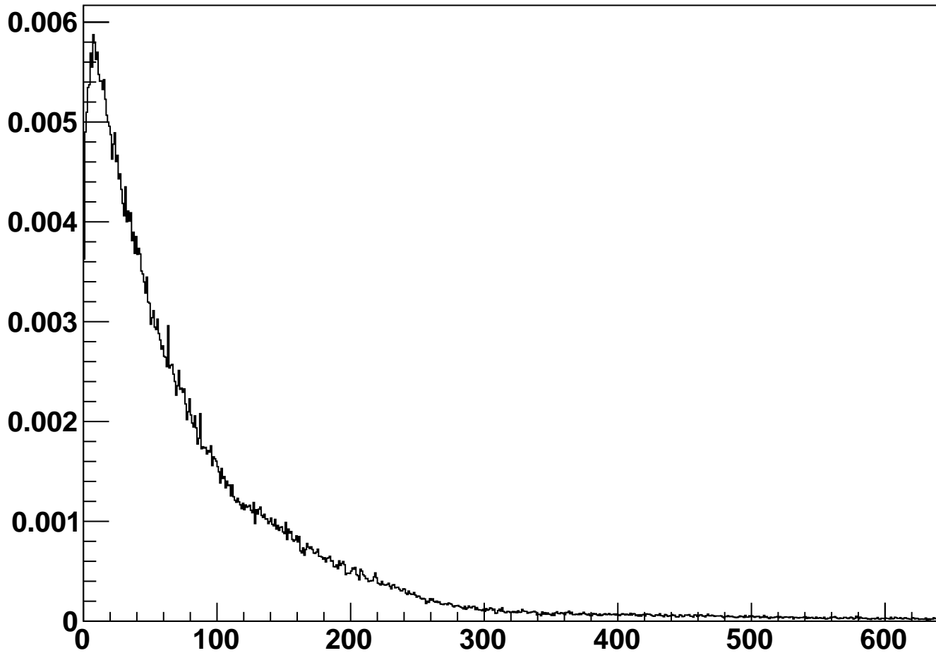
module_L3b_halfmodule_axial_sensor0 - Occupancy
