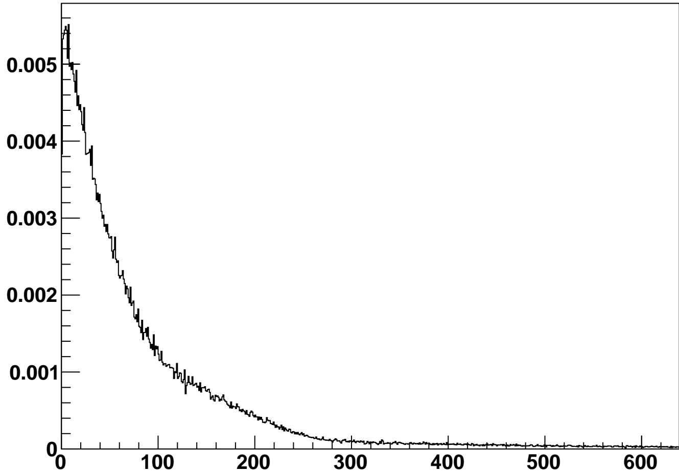
module_L3t_halfmodule_axial_sensor0 - Occupancy
