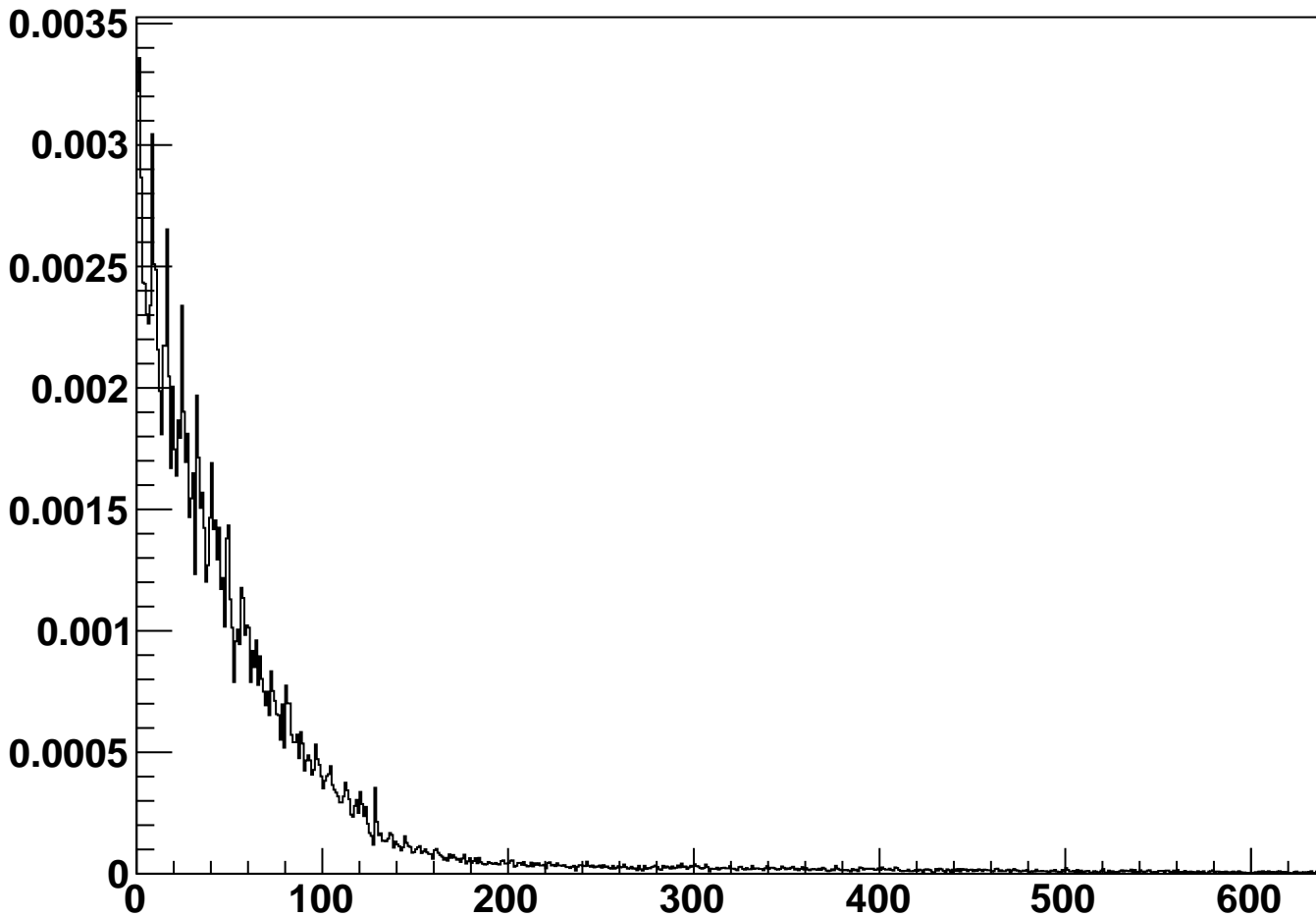
module_L2t_halfmodule_axial_sensor0 - Cluster Occupancy
