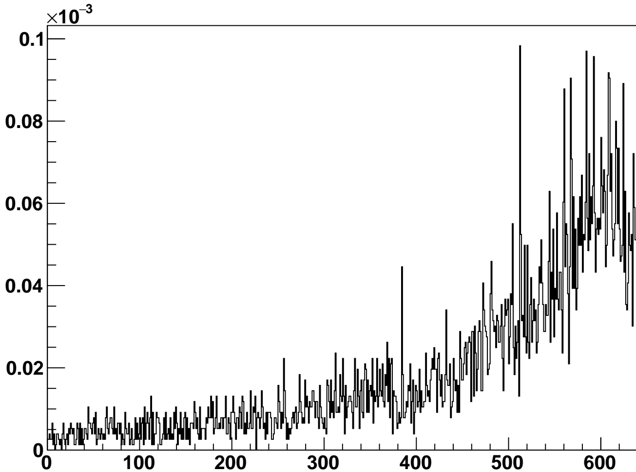
module_L6b_halfmodule_axial_slot_sensor0 - Cluster Occupancy
