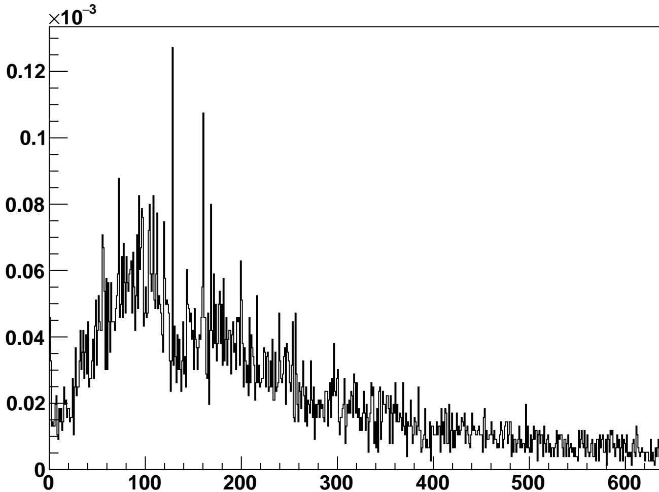
module_L6t_halfmodule_stereo_slot_sensor0 - Cluster Occupancy
