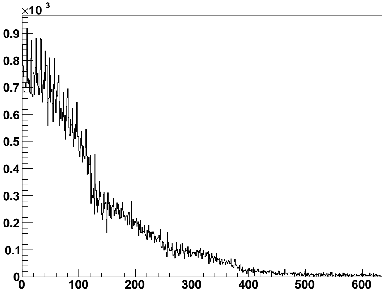
module_L4t_halfmodule_axial_hole_sensor0 - Cluster Occupancy
