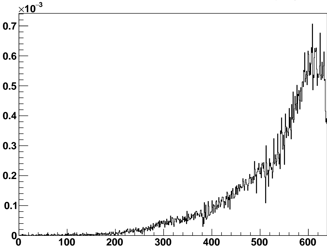
module_L4t_halfmodule_axial_slot_sensor0 - Cluster Occupancy
