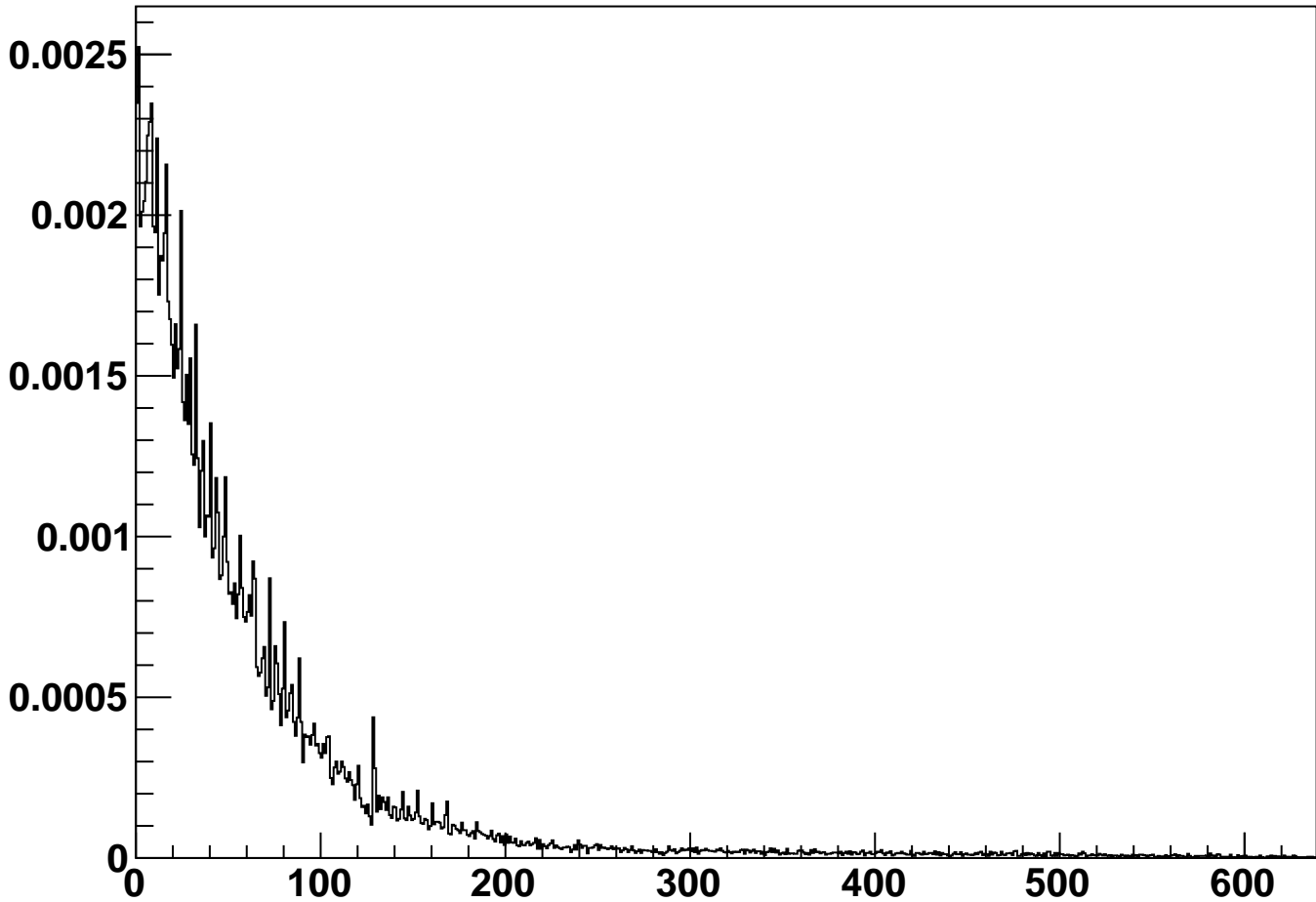
module_L2b_halfmodule_axial_sensor0 - Cluster Occupancy
