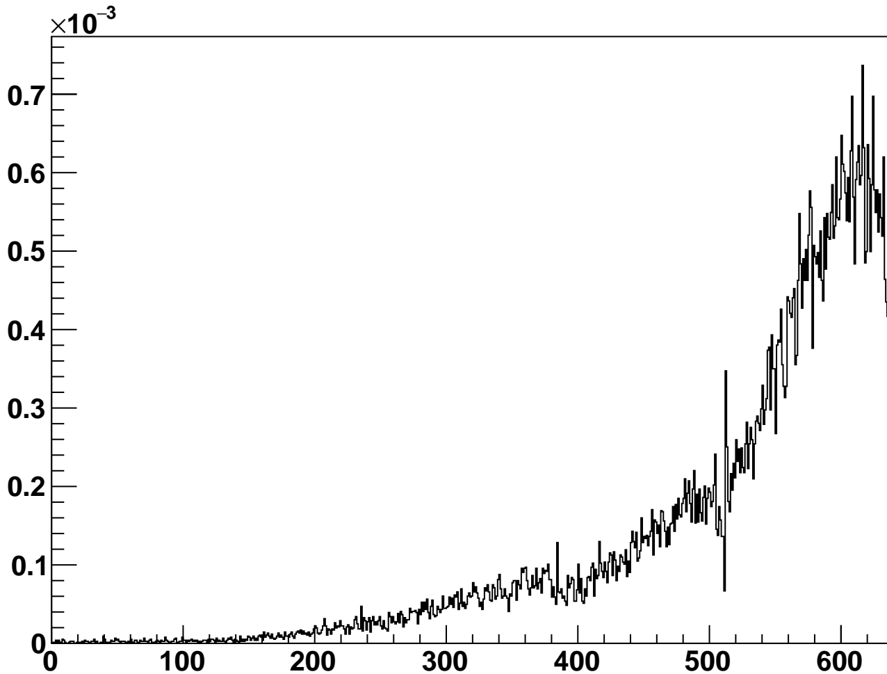
module_L4b_halfmodule_axial_slot_sensor0 - Cluster Occupancy
