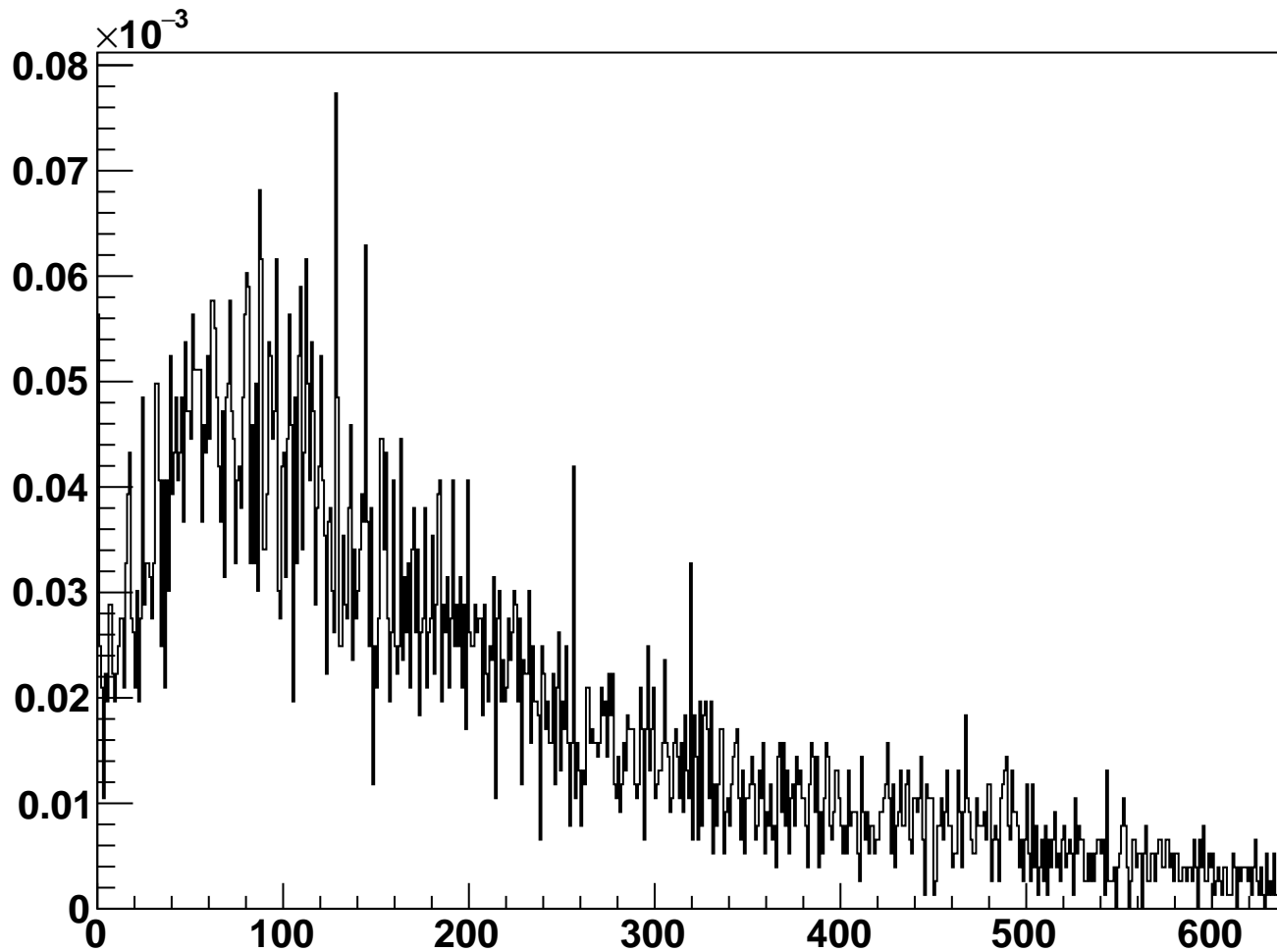
module_L5t_halfmodule_stereo_slot_sensor0 - Cluster Occupancy
