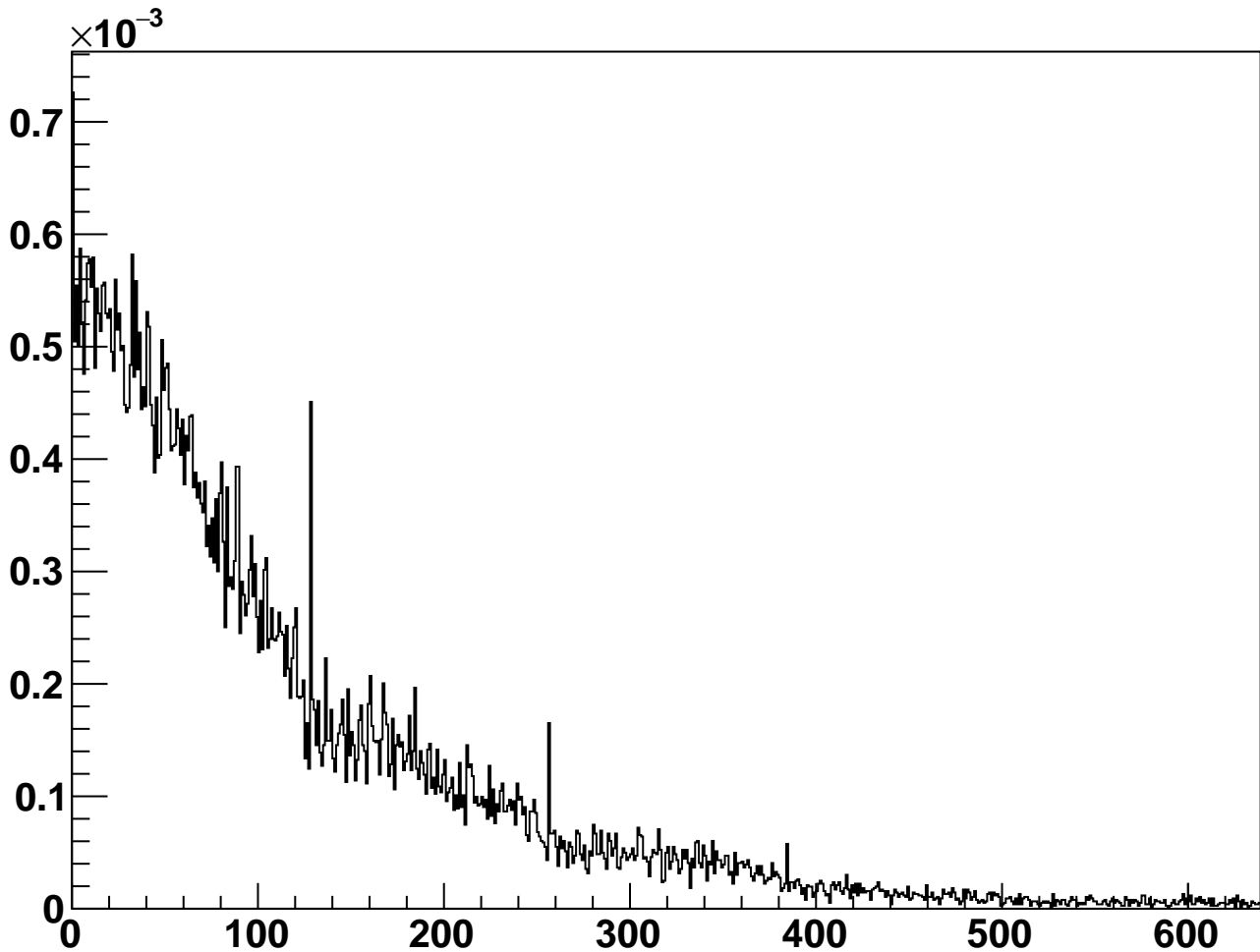
module_L4b_halfmodule_axial_hole_sensor0 - Cluster Occupancy
