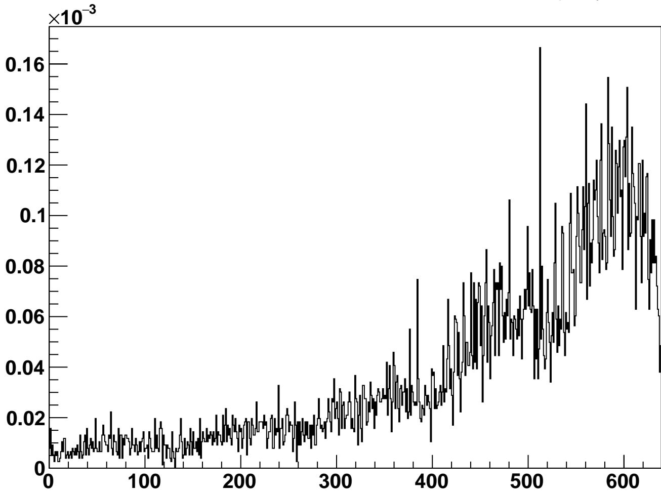
module_L6t_halfmodule_axial_slot_sensor0 - Cluster Occupancy
