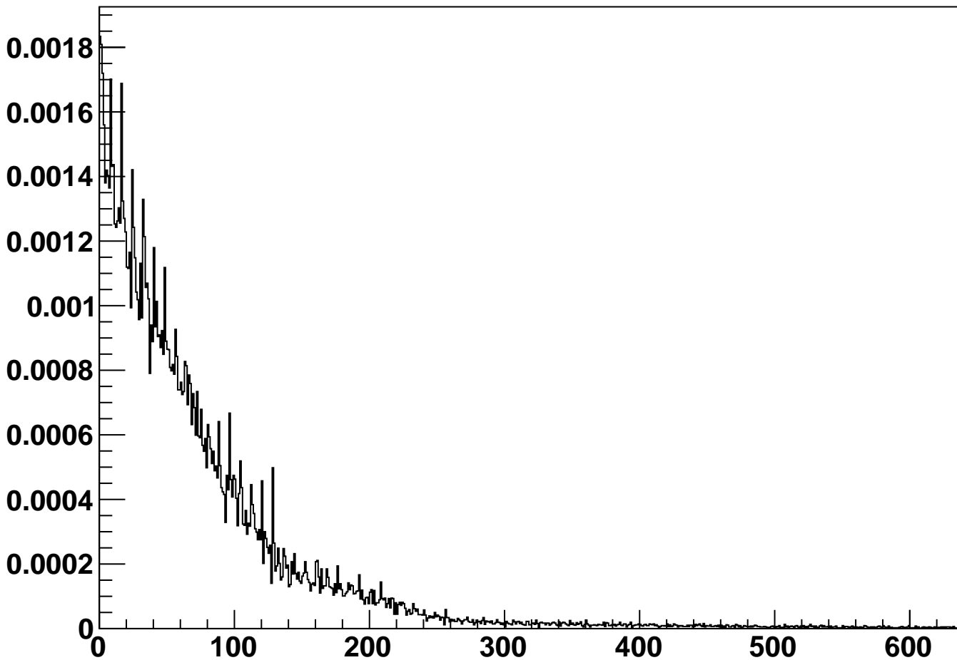
module_L3t_halfmodule_axial_sensor0 - Cluster Occupancy
