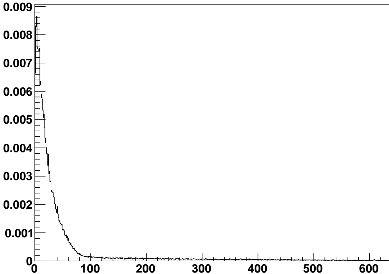
module_L1t_halfmodule_axial_sensor0 - Cluster Occupancy
