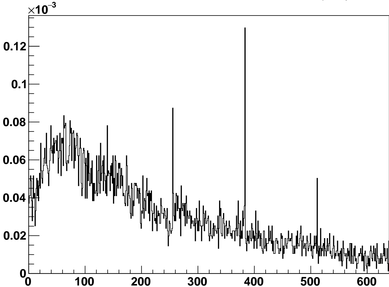
module_L6b_halfmodule_stereo_slot_sensor0 - Occupancy
