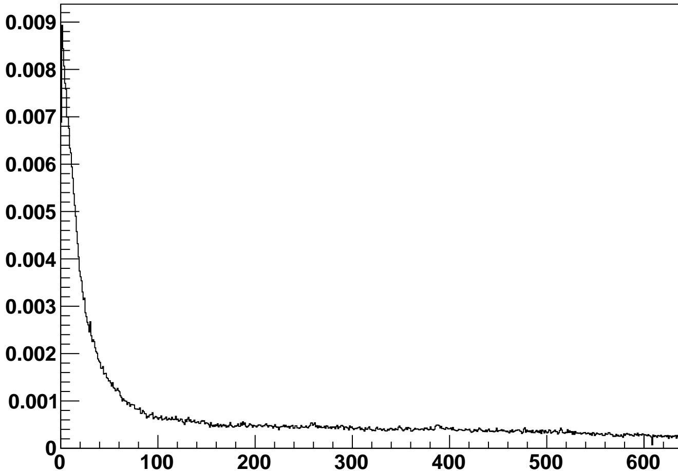
module_L1t_halfmodule_axial_sensor0 - Occupancy
