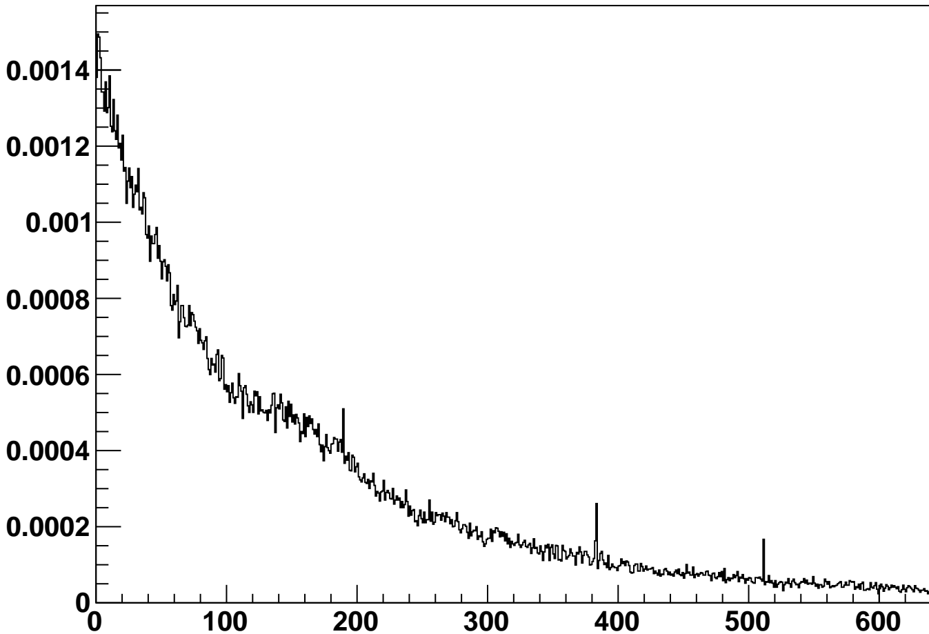
module_L6b_halfmodule_axial_hole_sensor0 - Occupancy
