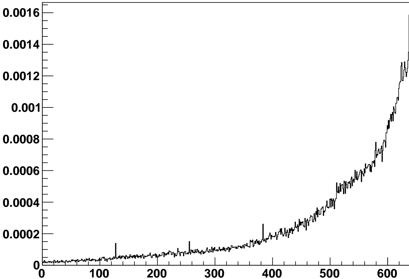
module_L5b_halfmodule_stereo_hole_sensor0 - Occupancy
