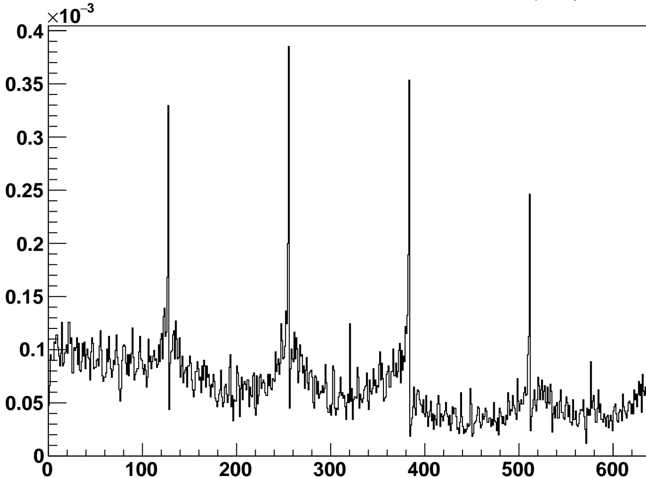
module_L6t_halfmodule_stereo_slot_sensor0 - Occupancy
