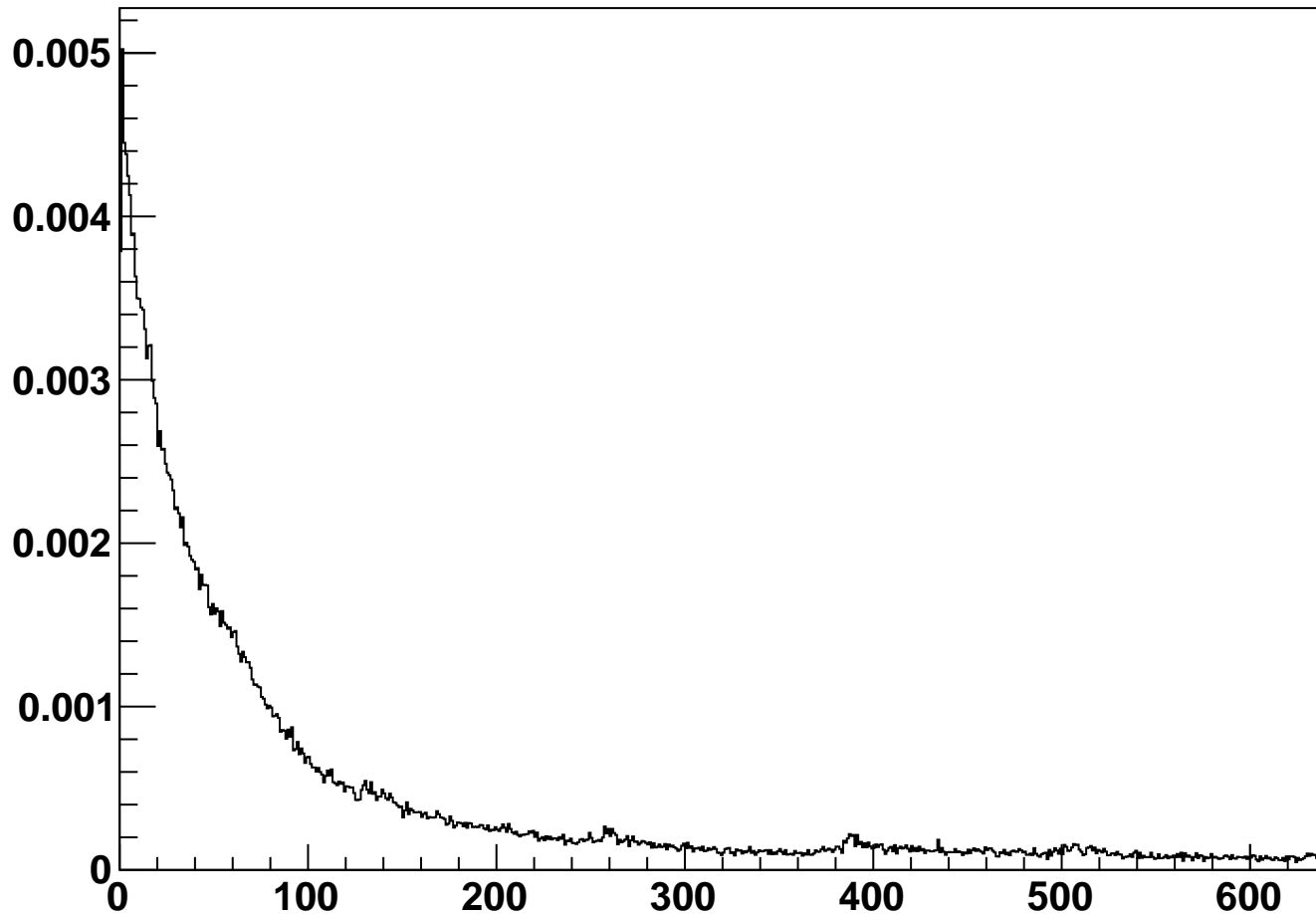
module_L3b_halfmodule_axial_sensor0 - Occupancy
