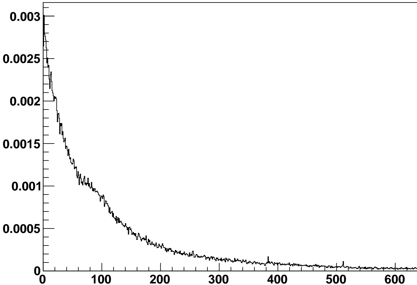
module_L4b_halfmodule_axial_hole_sensor0 - Occupancy
