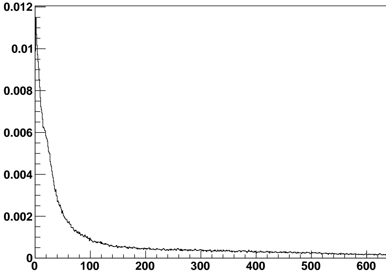
module_L1b_halfmodule_axial_sensor0 - Occupancy
