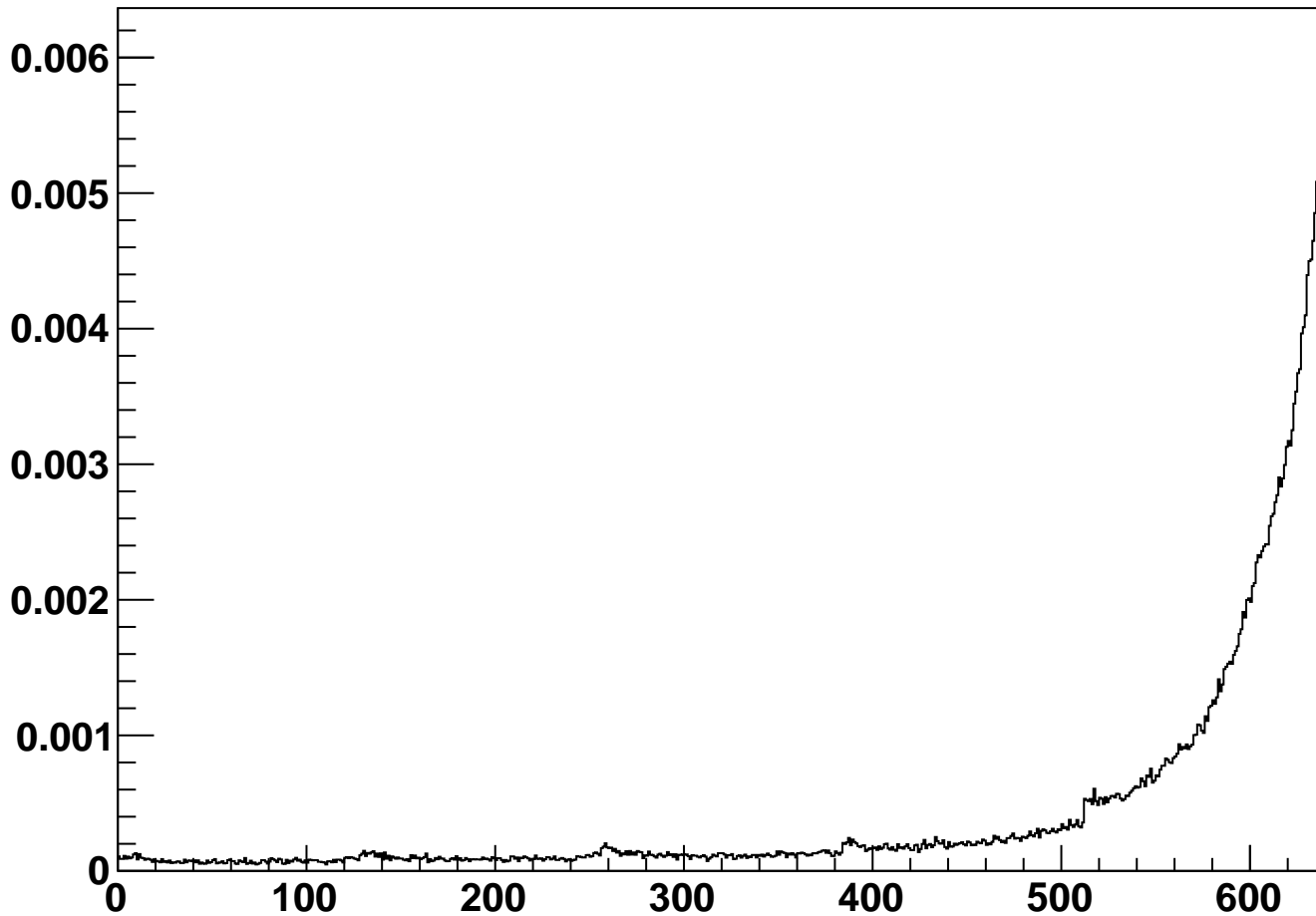
module_L2b_halfmodule_stereo_sensor0 - Occupancy
