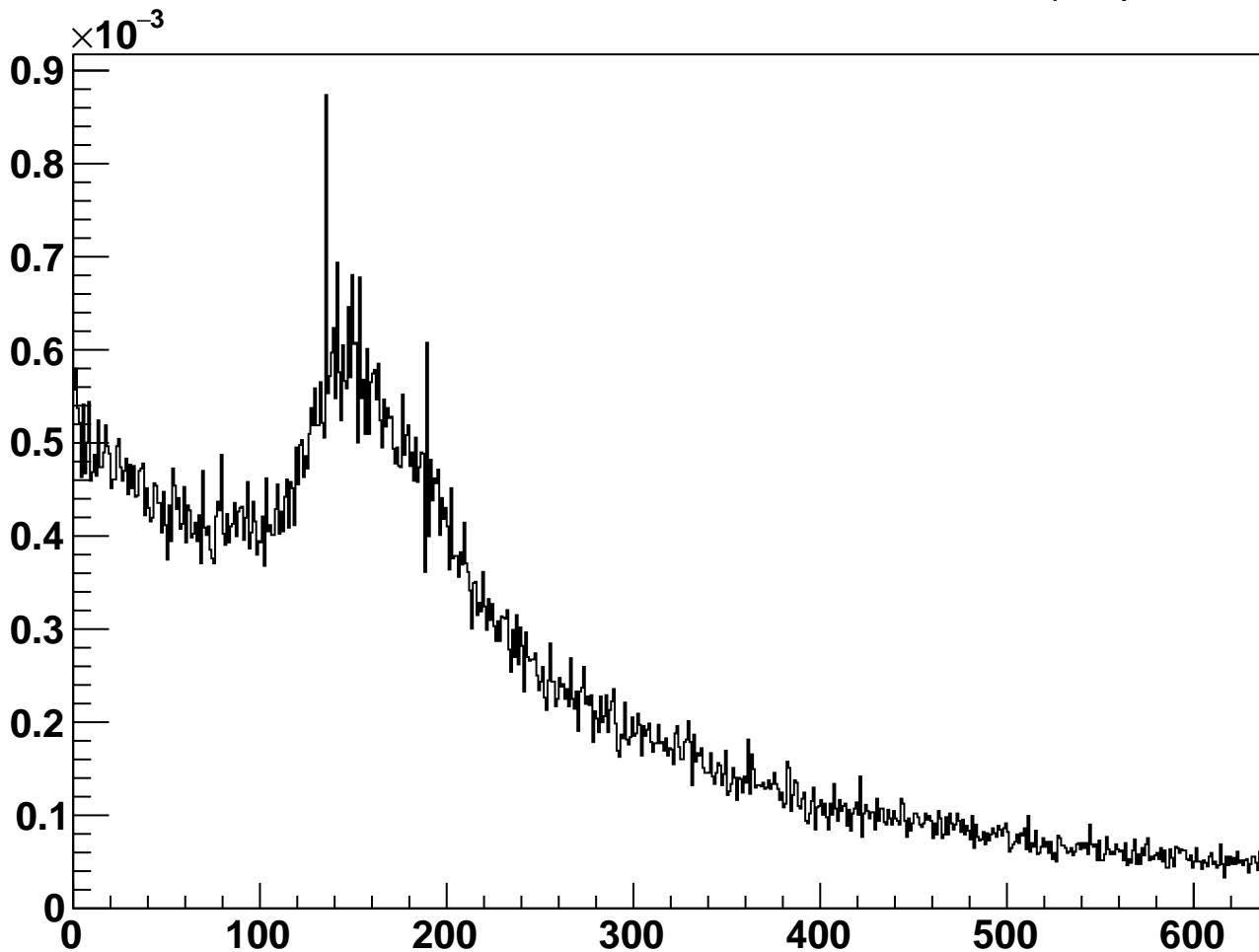
module_L6b_halfmodule_axial_hole_sensor0 - Cluster Occupancy
