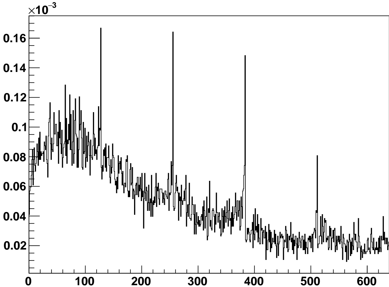
module_L6t_halfmodule_stereo_slot_sensor0 - Cluster Occupancy
