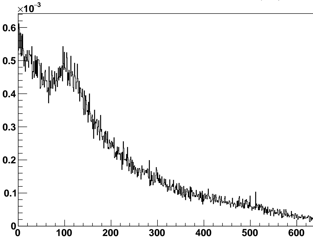
module_L5t_halfmodule_axial_hole_sensor0 - Cluster Occupancy
