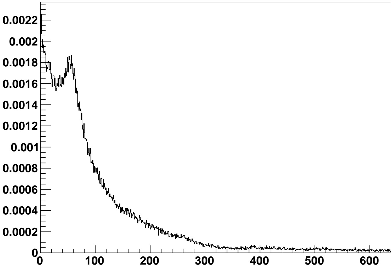
module_L3b_halfmodule_axial_sensor0 - Cluster Occupancy
