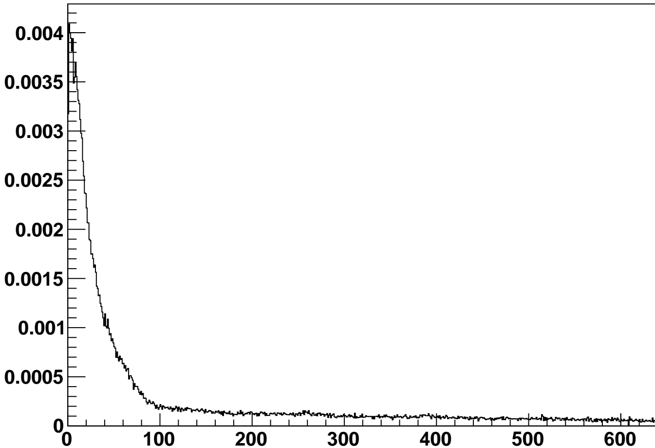
module_L1t_halfmodule_axial_sensor0 - Cluster Occupancy
