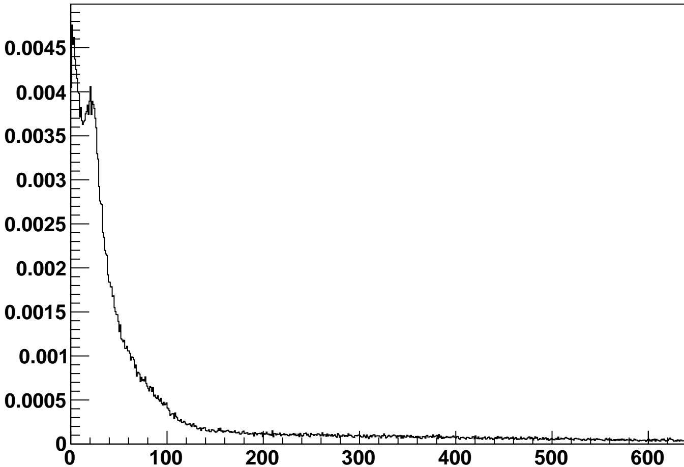
module_L1b_halfmodule_axial_sensor0 - Cluster Occupancy
