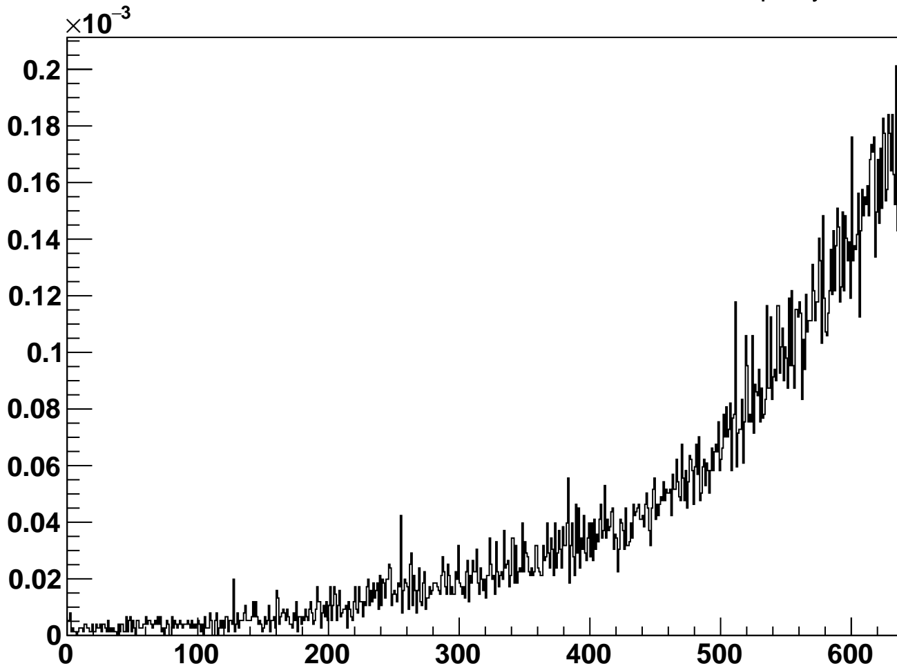
module_L4t_halfmodule_axial_slot_sensor0 - Cluster Occupancy
