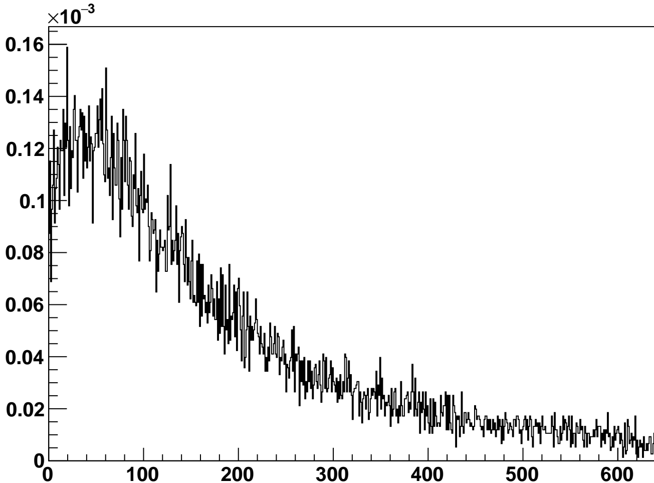
module_L5t_halfmodule_stereo_slot_sensor0 - Cluster Occupancy
