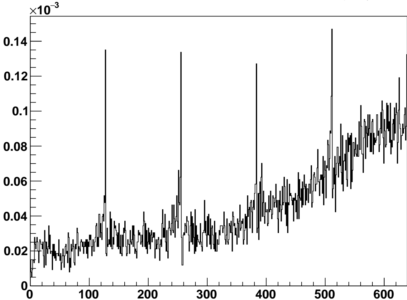
module_L6t_halfmodule_axial_slot_sensor0 - Cluster Occupancy
