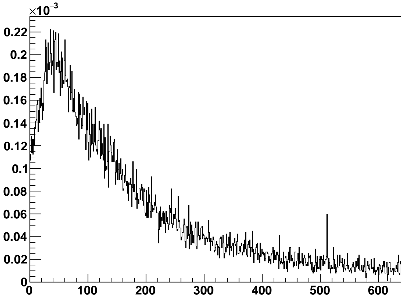
module_L5b_halfmodule_stereo_slot_sensor0 - Cluster Occupancy
