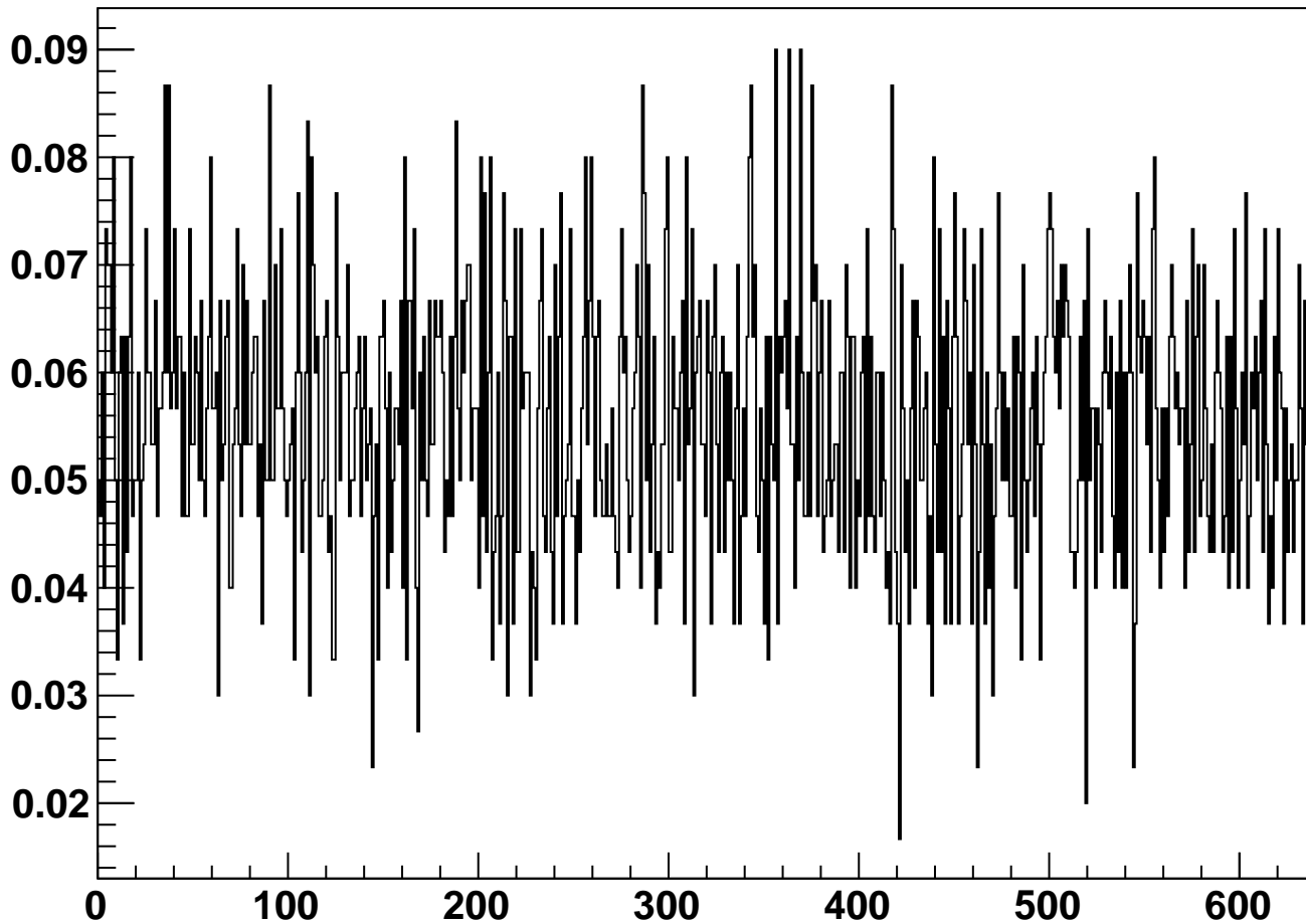
module_L3t_halfmodule_axial_sensor0 - Occupancy
