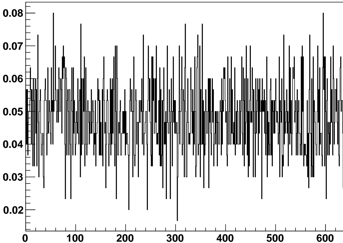
module_L3b_halfmodule_stereo_sensor0 - Occupancy
