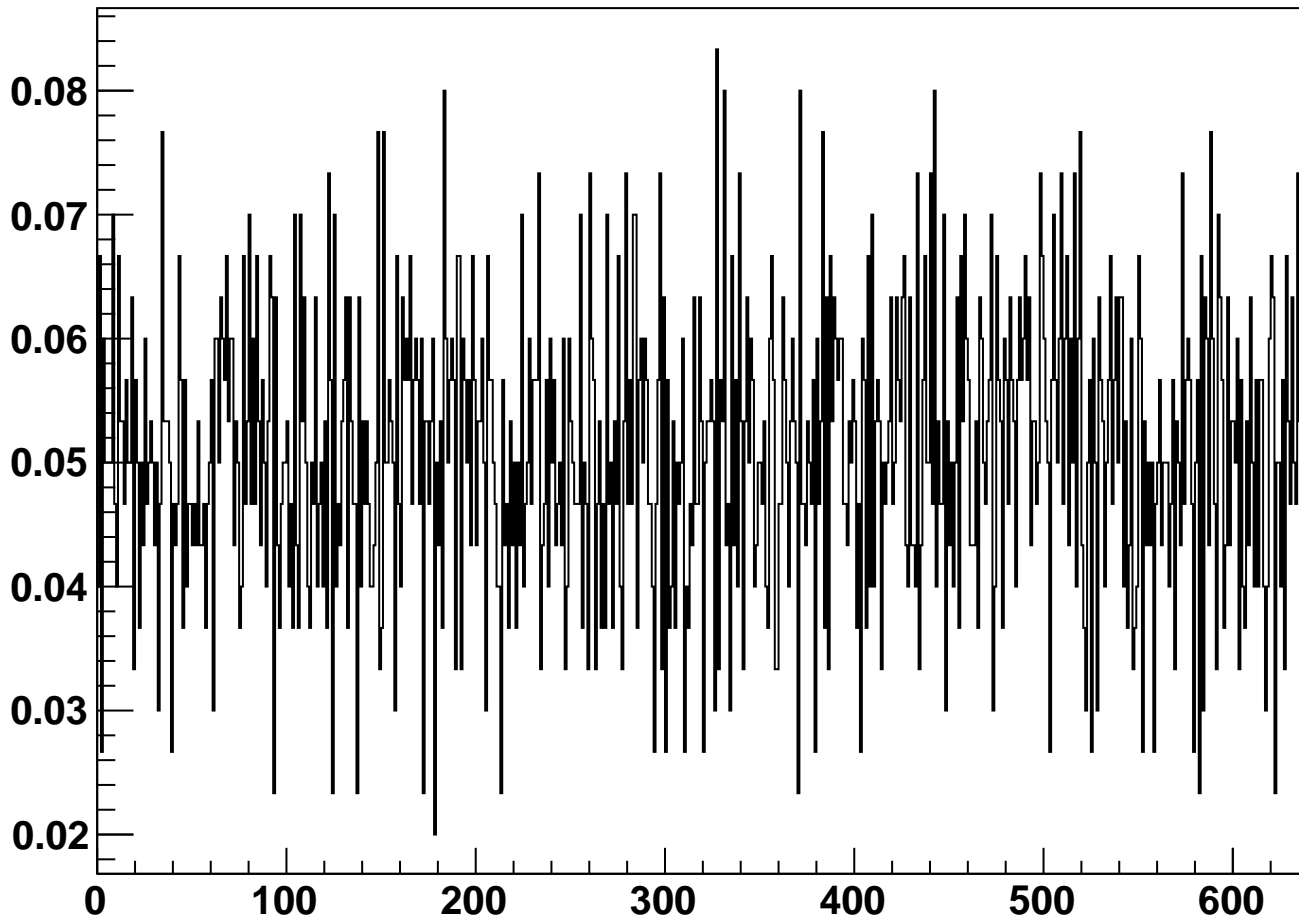
module_L5b_halfmodule_stereo_hole_sensor0 - Occupancy
