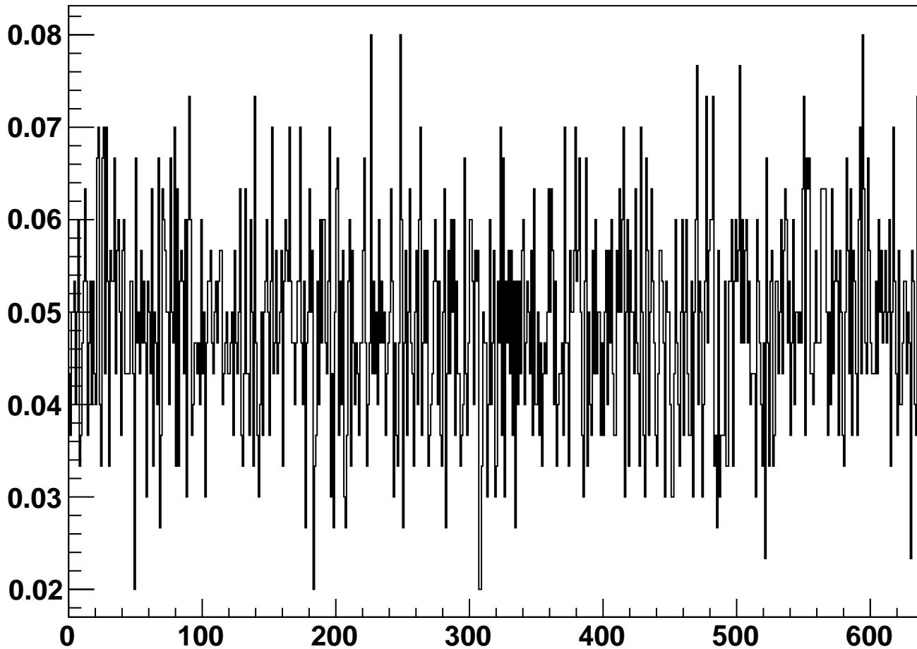
module_L6b_halfmodule_stereo_slot_sensor0 - Occupancy
