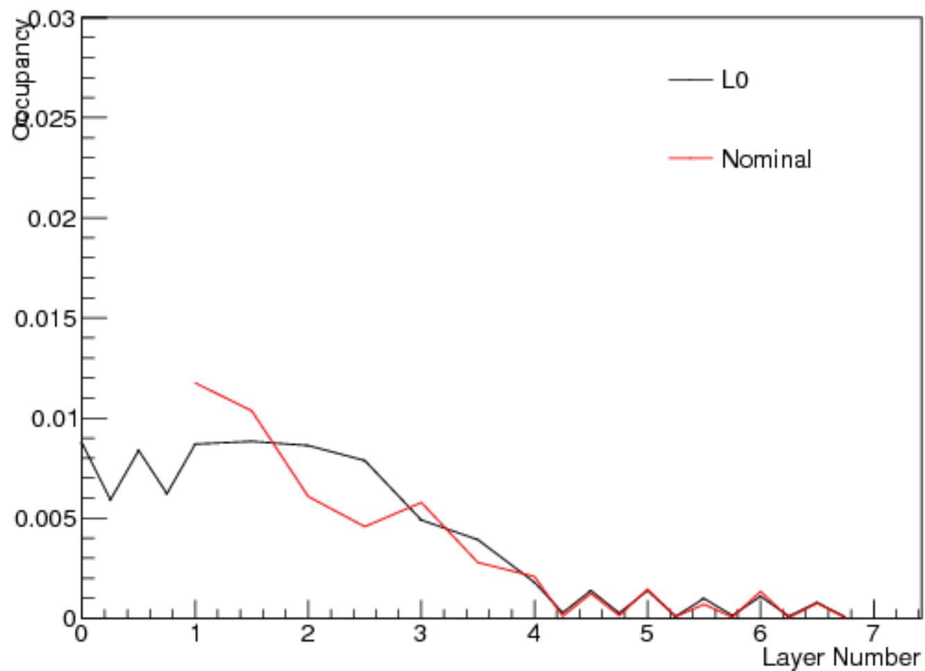
SVT Sensor Edge Cluster Occupancies Top
