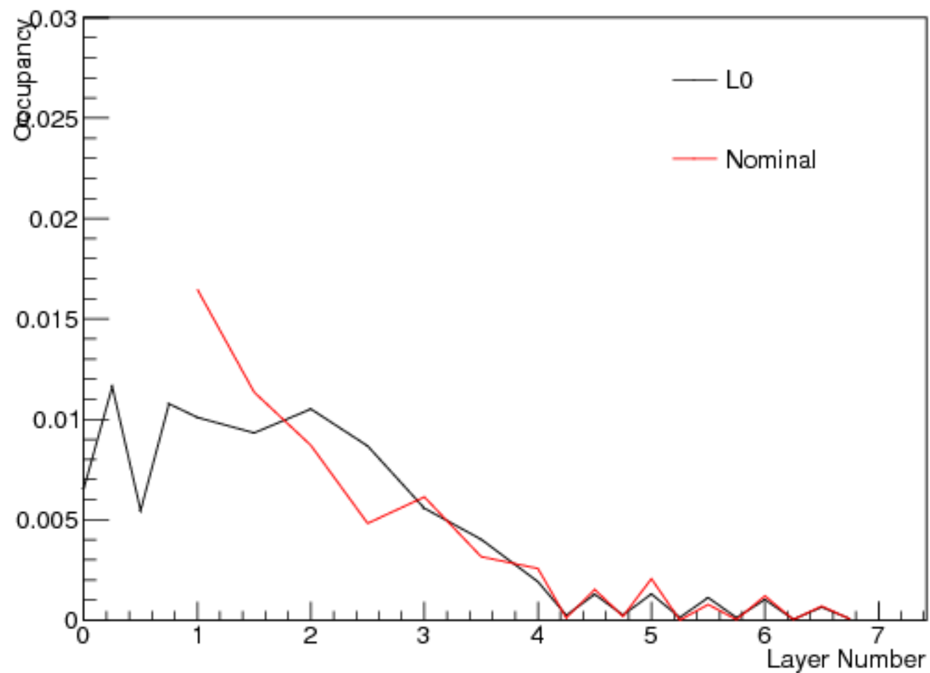
SVT Sensor Edge Cluster Occupancies Bottom
