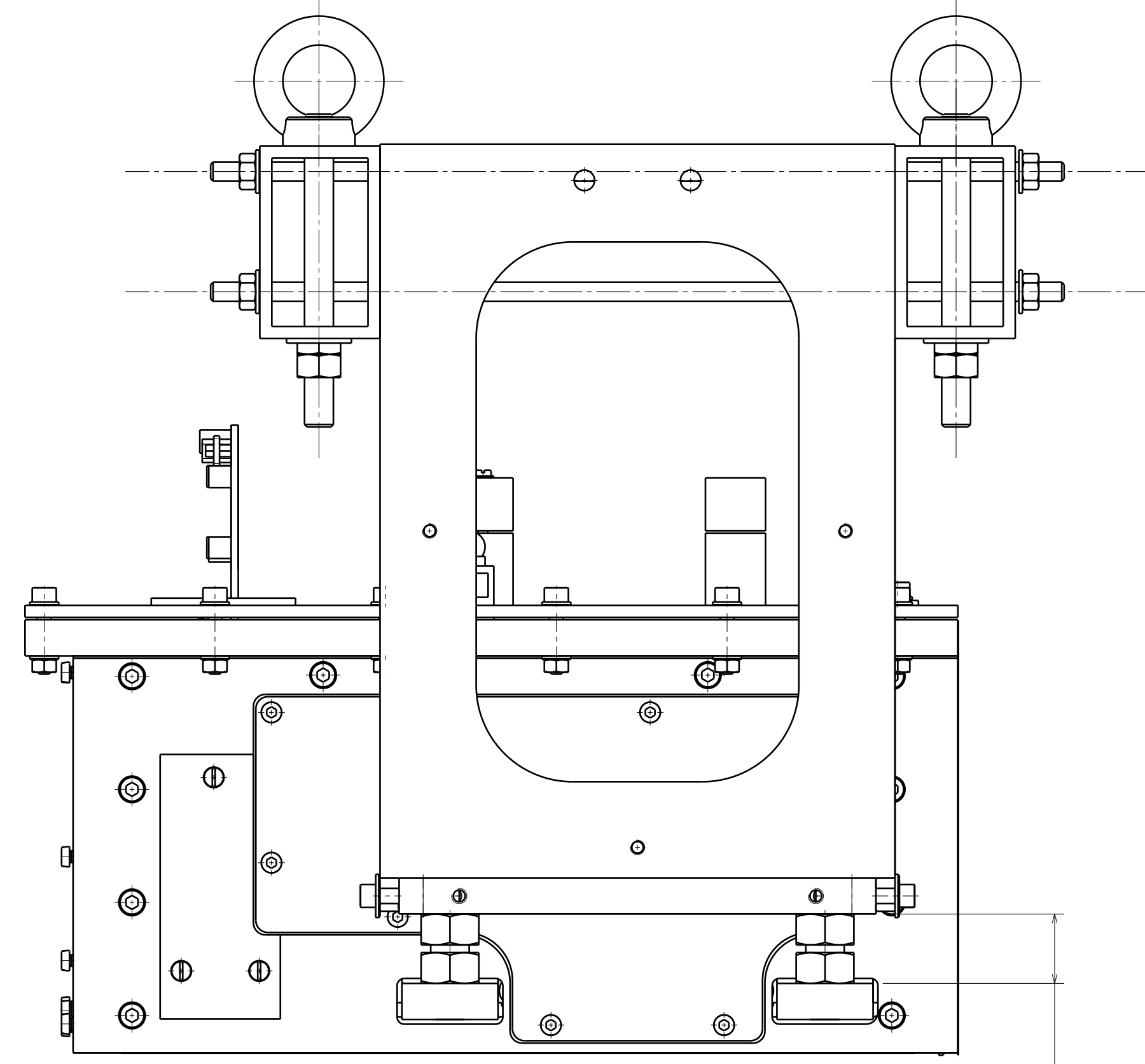
Vue de droite Echelle : 1:2
