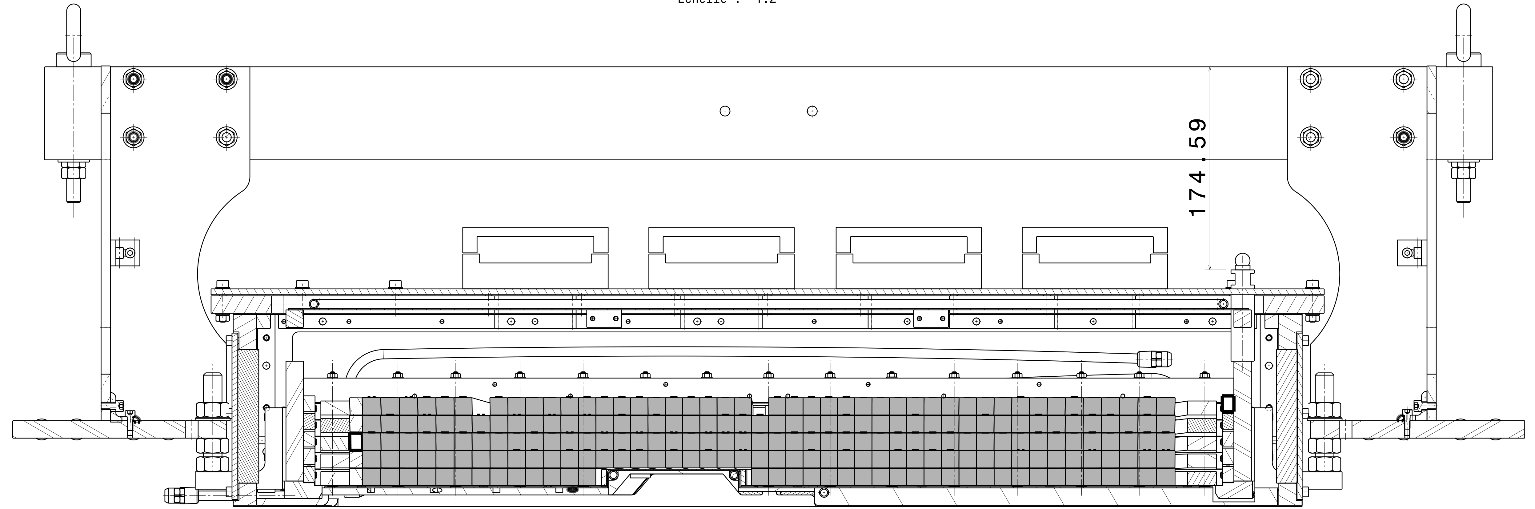
Coupe A-A Echelle : 1:2
