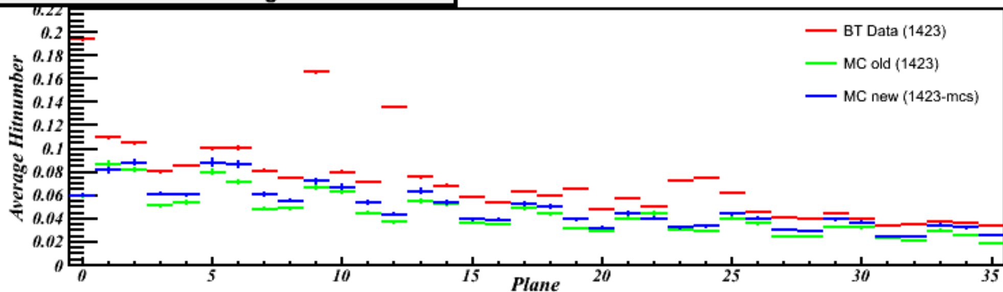
Protons 6 GeV/c 0 deg -- TWR 2
