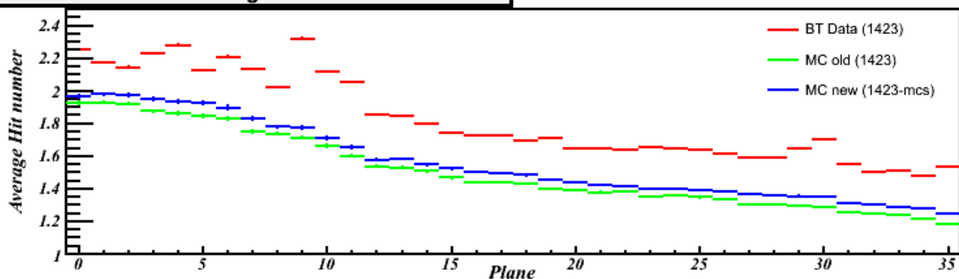
Protons 6 GeV/c 0 deg -- TWR 2 + TWR 3
