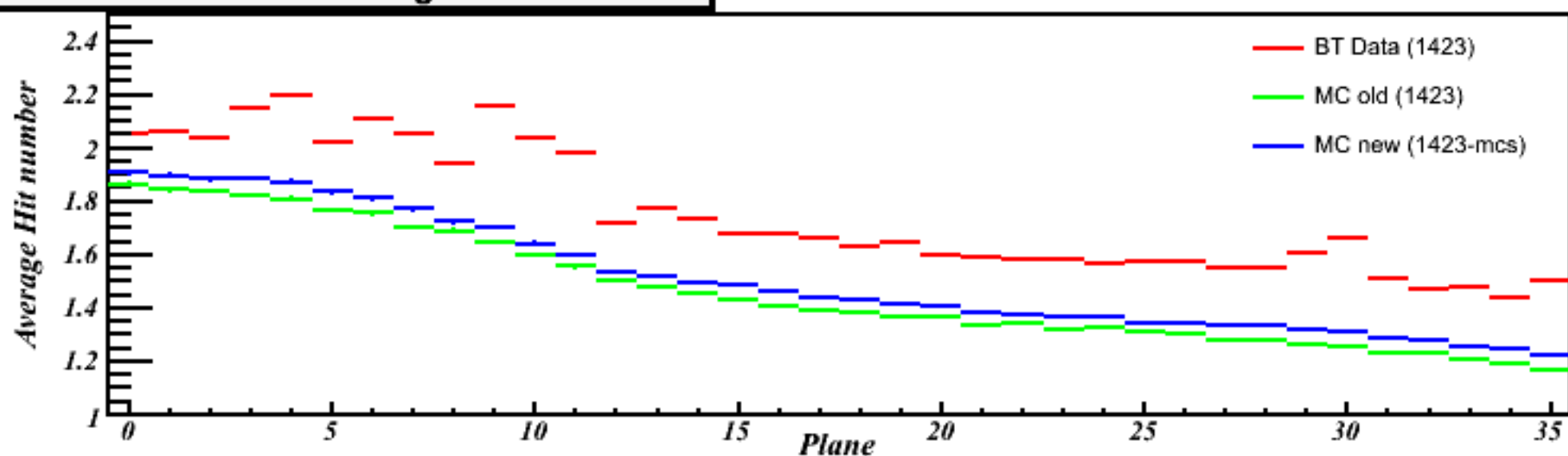
Protons 6 GeV/c 0 deg -- TWR 3
