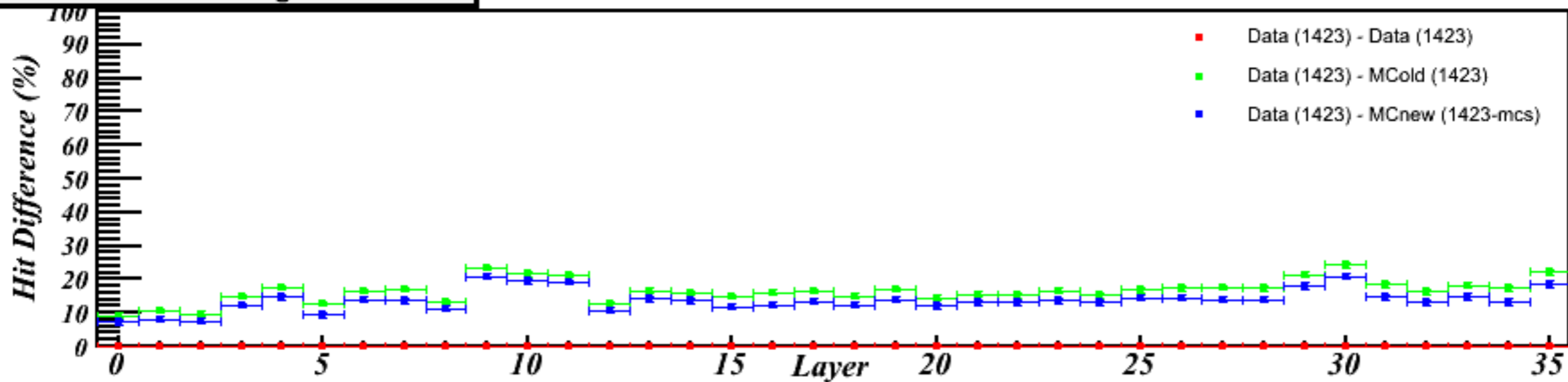
Protons 6 GeV/c 0 deg -- TWR 3
