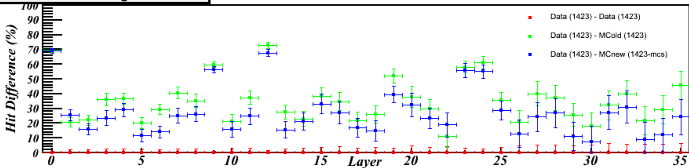
Protons 6 GeV/c 0 deg -- TWR 2
