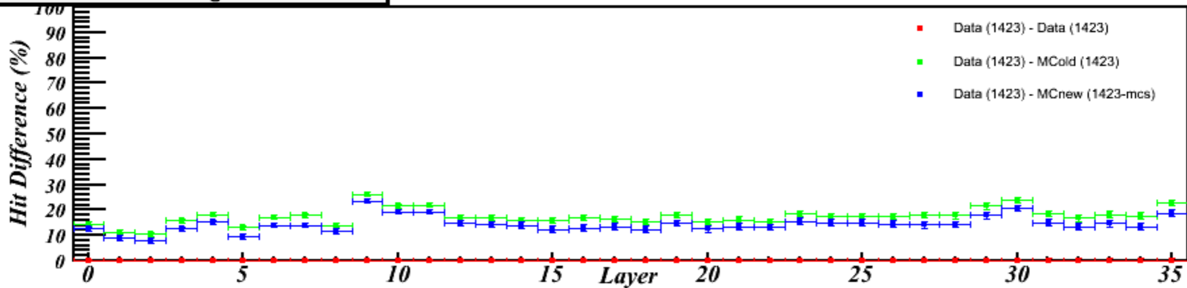
Protons 6 GeV/c 0 deg -- TWR 2+3
